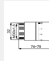
Mesures de la tête thermostatique
