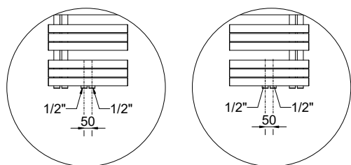
Détail de l'entraxe central (collecteurs à gauche)
