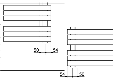
Mesures pour robinets de type Kristal
