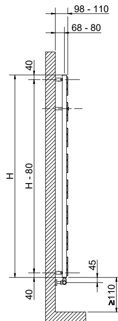
Mesures pour robinets de type Kristal
