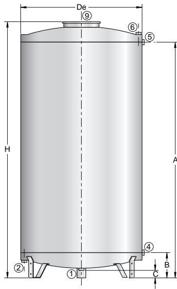
PASSO D'UOMO CENTRATO SULL'ASSE PER MODELLI DA 125 A 2000
