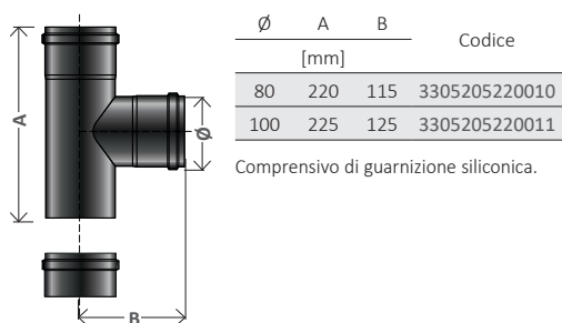
Fig. 11 Raccordo a T 90° FEMMINA-FEMMINA-MASCHIO con tappo cieco
