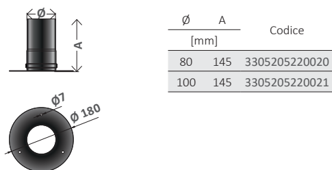
Fig. 9 Rosone ∅ 180 con elemento
