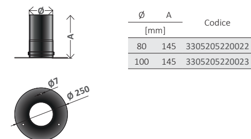
Fig. 10 Rosone ∅ 250 con elemento
