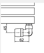
Misure per valvola kristal corner con testa termostatica
